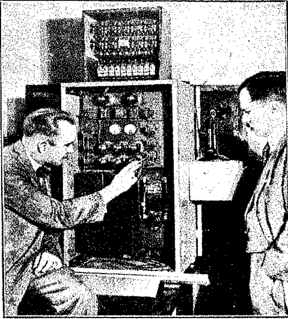
صورة الجهاز الكهربائي للسيد « الرجل الميكانيكي » الذي يطبع صوت الانسان وينفذ اوامره . وقد وقف امامه مخترعه المستر ونسلي الامبريكي يشرح لبعض الزائرين سر تركيبه العجيب
